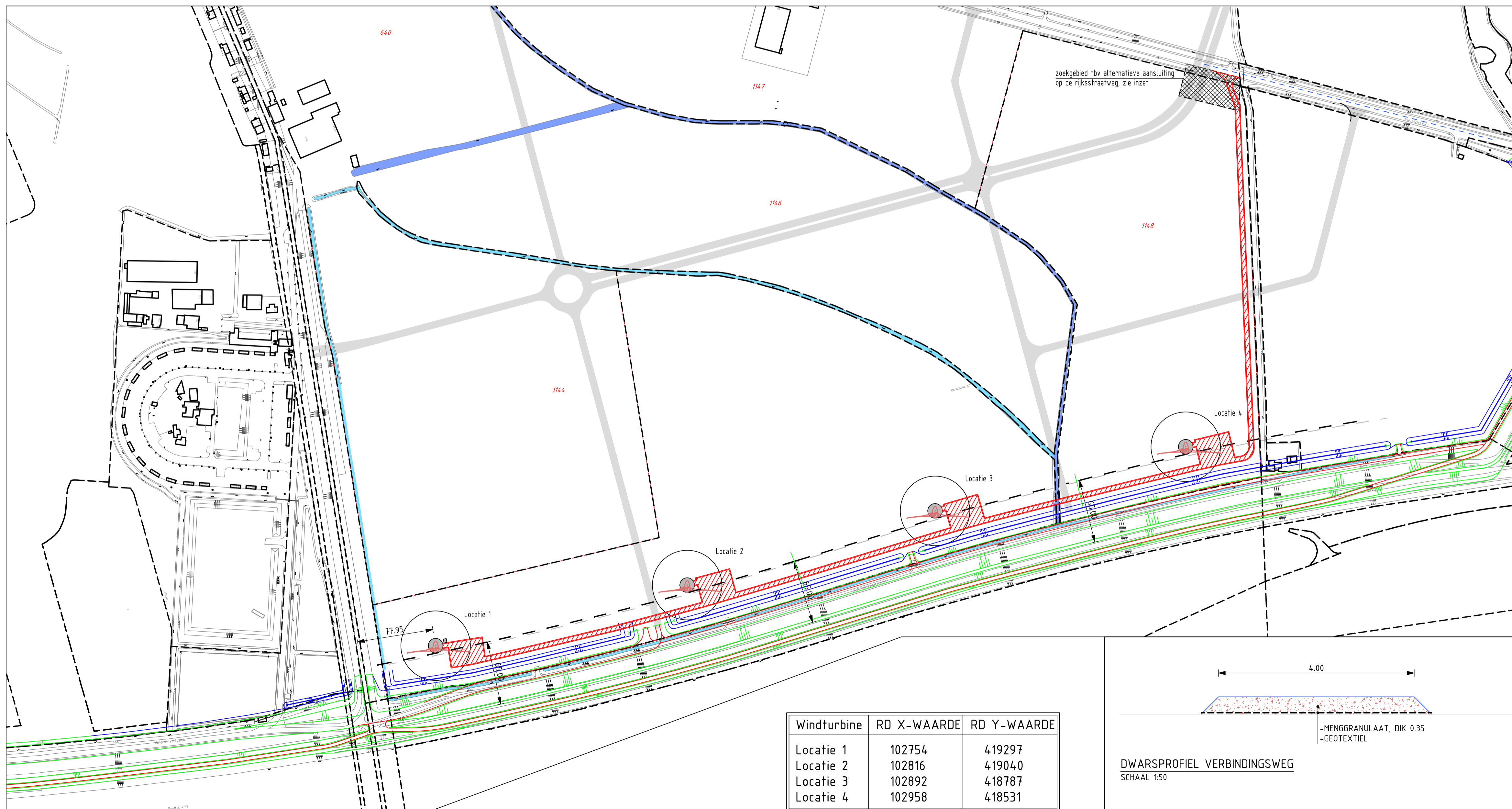
DETAILAANSLUITING RIJKSSTRAATWEG SCHAAL 1:500
