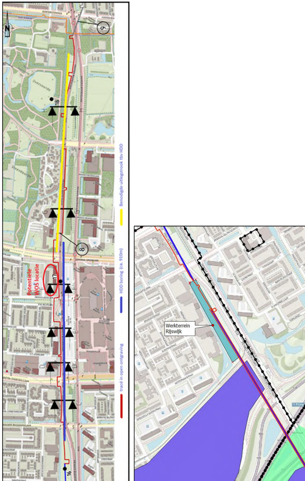
Afbeelding 1.3. Tracéwijziging mei 2019: extra HDD-boring (blauwe lijn) tussen Brederodelaan en Generaal Spoorlaan (910 m) en de locatie van het werkkerrein in Rijswijk.
