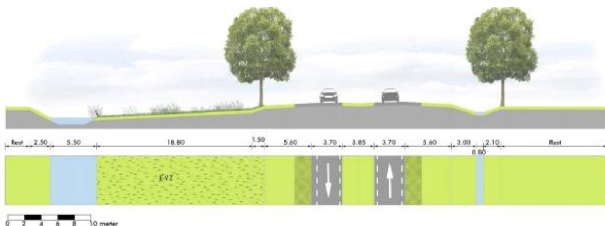
Figuur 3.21 Profiel EVZ
