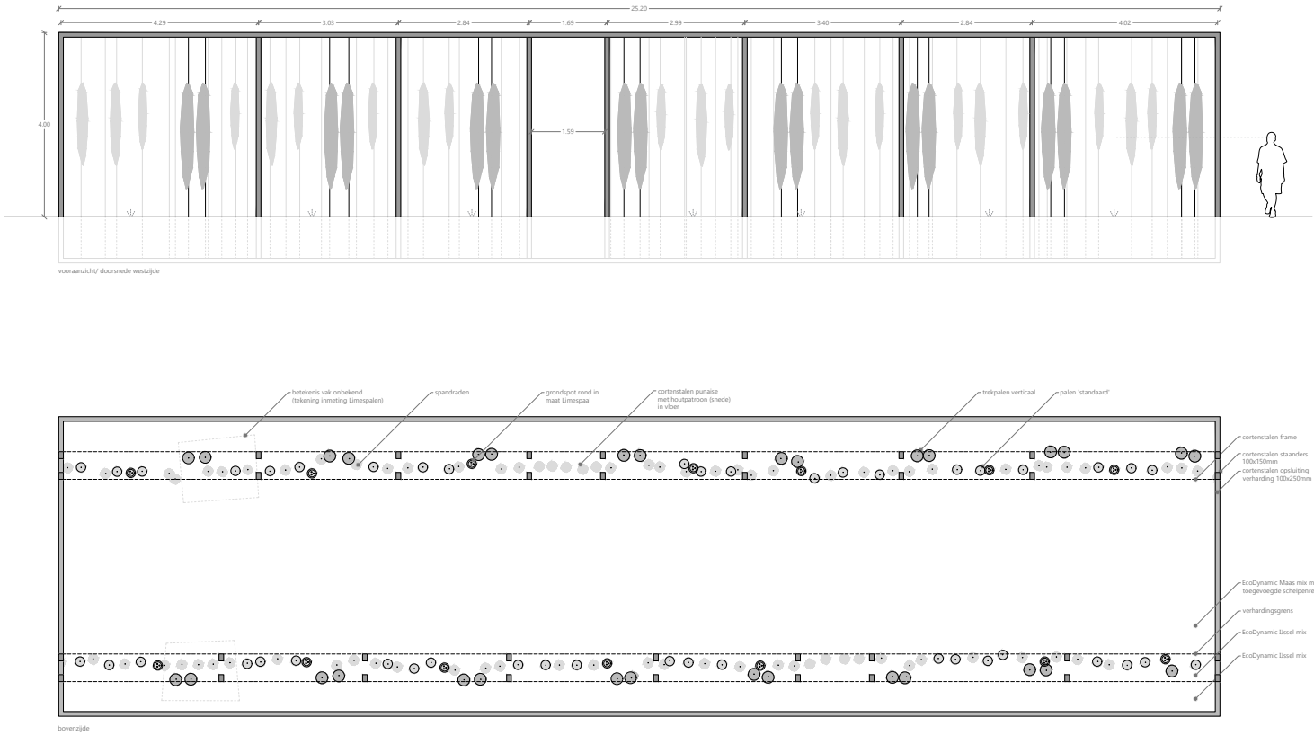
Schetsontwerp BoschSlabbers voor het Limes monument
