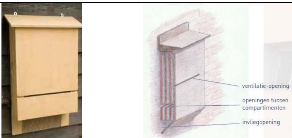
Figuur 3.27 Vleermuiskast Vivara (afmetingen 51 x 16,5 x 78 centimeter) en een doorsnede daarvan (rechts).
