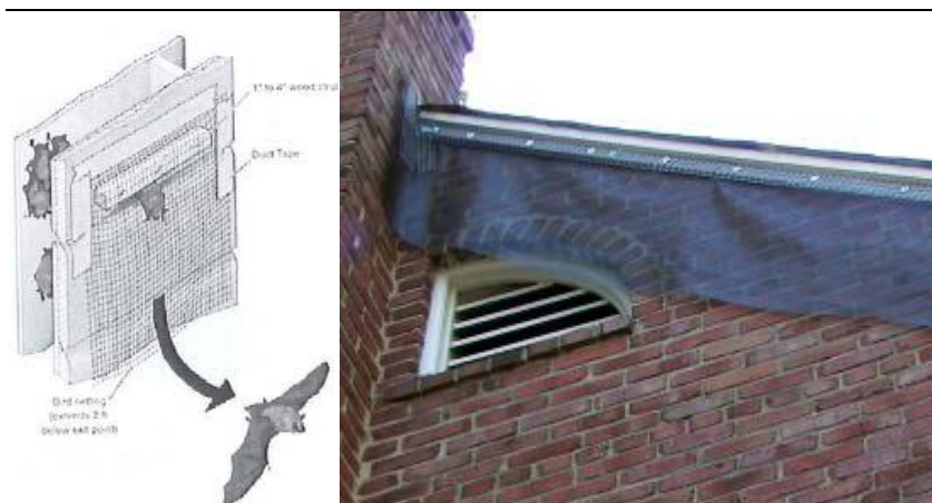
Figuur 3.28 'Exclusion flaps' voor vleermuizen.
