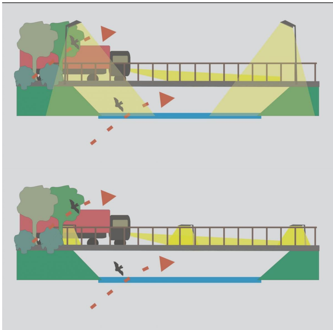
Figuur 3.11 Voorkom verstrooiing van licht vanaf de bovenzijde van het brugdek door de verlichting lager aan te brengen (Zoogdiervereniging, 2012).
