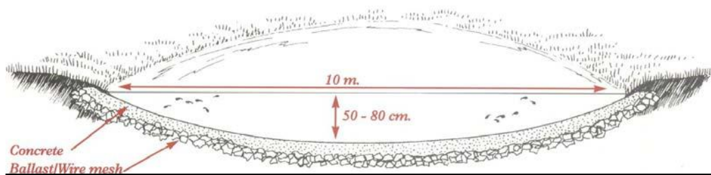
Figuur 3.30 Betonnen schotel geschikt als voortplantingshabitat voor de rugstreppad.
