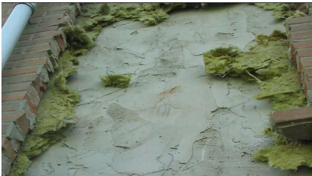
Figuur 3.18 Blootgelegde spouwmuur waar ook het isolatiemateriaal is verwijderd.
