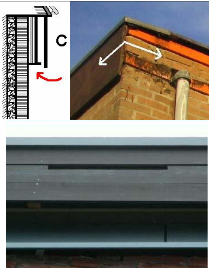
Figuur 3.22 Varianten van gevelbetimmering als verblijfplaats voor vleermuizen.
