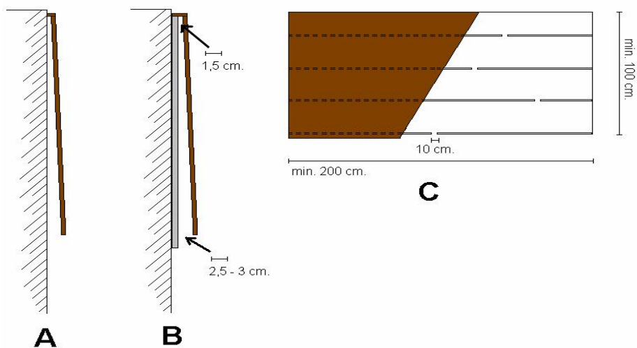
Figuur 3.21 Voorbeelden van gevelbetimmering geschikt als verblijfplaats voor vleermuizen.
