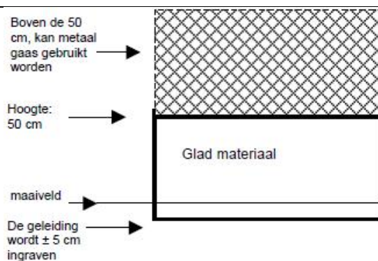
Figuur 3.31 Voorbeeld van de opbouw van een amfibiescherm (NB: diepte tot waarop het scherm wordt ingegraven staat hier foutief weergegeven).
